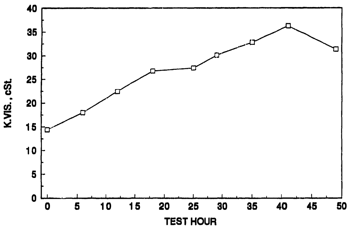
Figure F-2. AIPS-6, AL-19372, K. vis., 100°C
