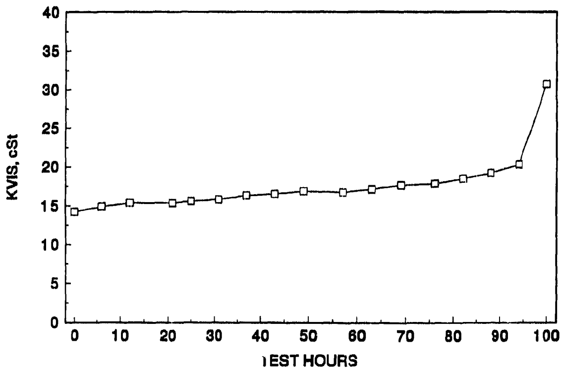
Figure E-2. AIPS-5, AL-19347, K. vis., 100°C
